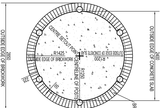
PLAN BASE SETOUT
