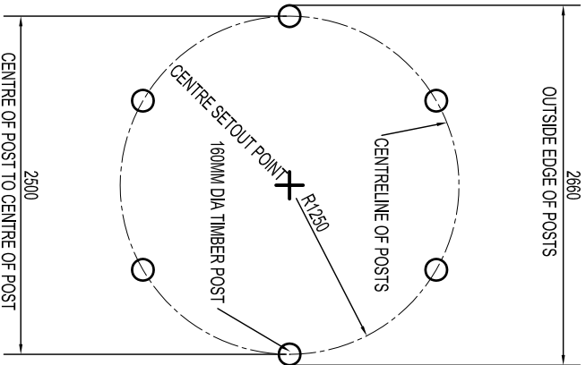
PLAN POST SETOUT
