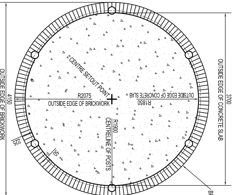
PLAN BASE SETOUT
