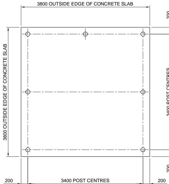
PLAN BASE SETOUT
