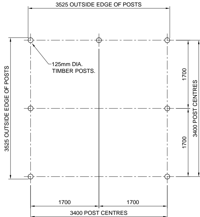
PLAN POST SETOUT
